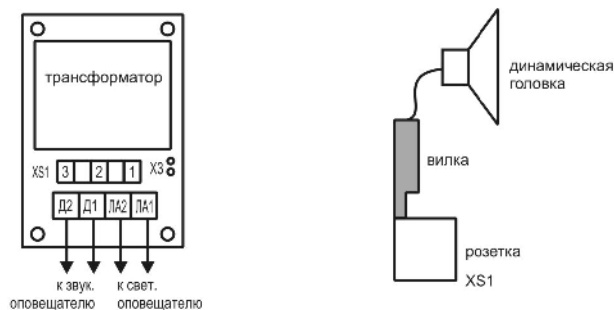
Рис. 1. Внешний вид платы динамической подключений
